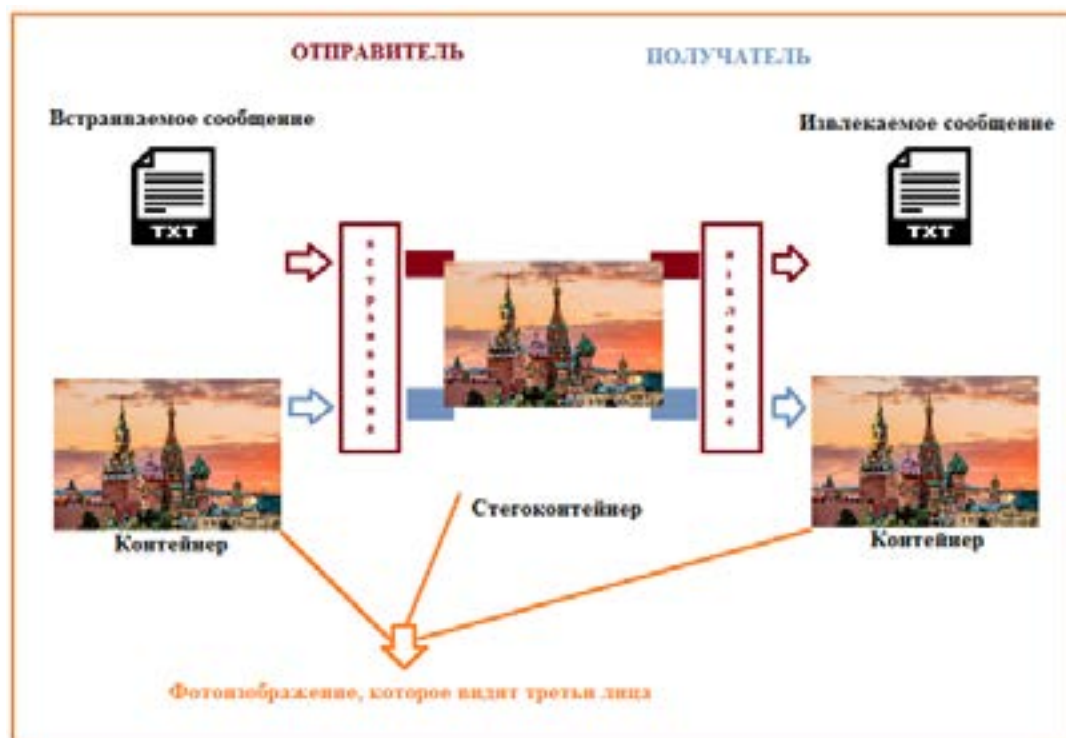
Рис. Стеганографический способ сокрытия текста
